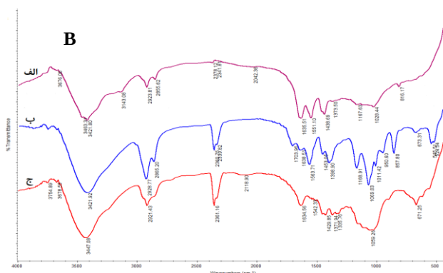
شکل ۱: آنالیز طیف سنجی مادون قرمز تبدیل فوری ناتامایسین (A) و آمفوتریسین B (B). فیلم نانوسولز باکتریایی (الف)، داروی ناتامایسین / آمفوتریسین B (ب)، فیلم نانوسولز اصلاح شده با دارو (ج).
